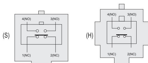
Konfiguracija kontakata
